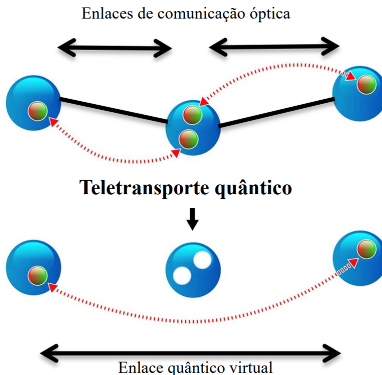
Figura 1. Enlace quântico virtual - EQV
